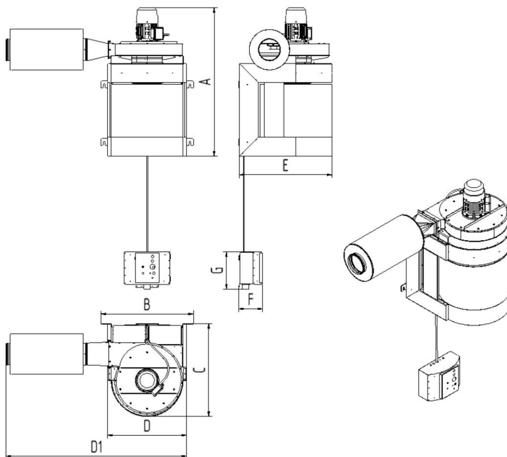
Abb. 17: Maßblatt
