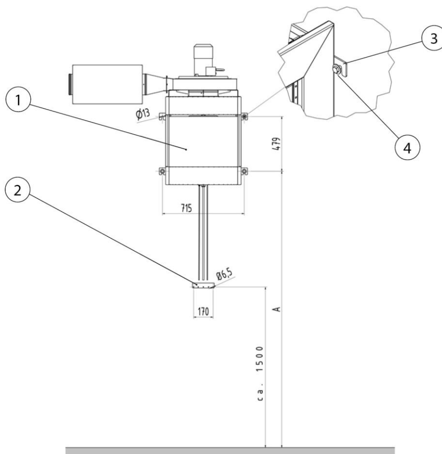
Abb. 7: Montagehöhe bestimmen
