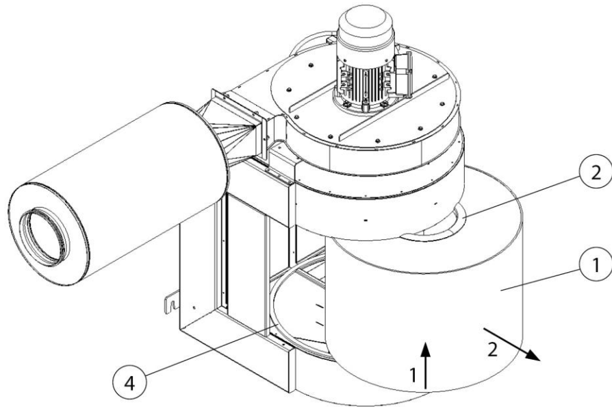
Abb. 13: Filterwechsel durchführen
